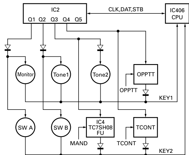
Fig. 14 Key input
